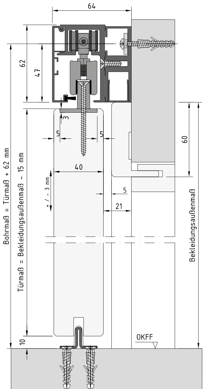
Montage mit Holztür vor Zarge
