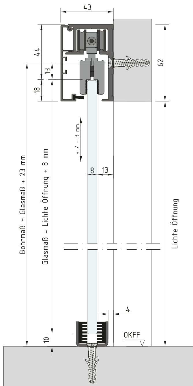
Montage mit Ganzglastür
