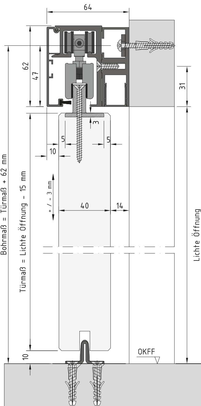
Montage mit Holztür
