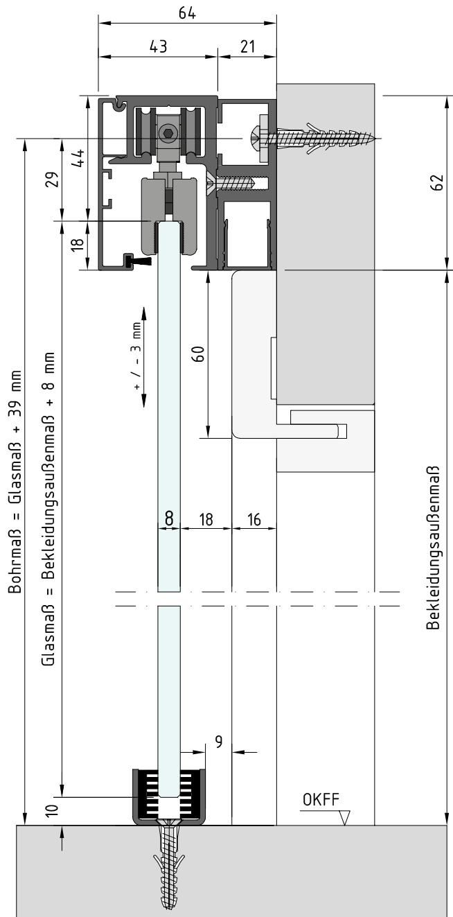
Montage mit Ganzglastür vor Zarge
