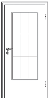
DIN LA / SP1 Friese: 160 mm Sockel: 400 mm
