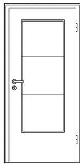
DIN LA / SP20 Friese: 160 mm Sockel: 400 mm
