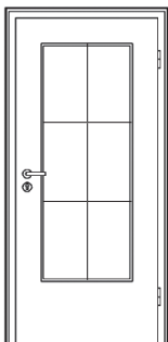
DIN LA / SP2 Friese: 160 mm Sockel: 400 mm
