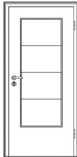
DIN LA / SP30 Friese: 160 mm Sockel: 400 mm
