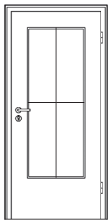
DIN LA / SP0 Friese: 160 mm Sockel: 400 mm
